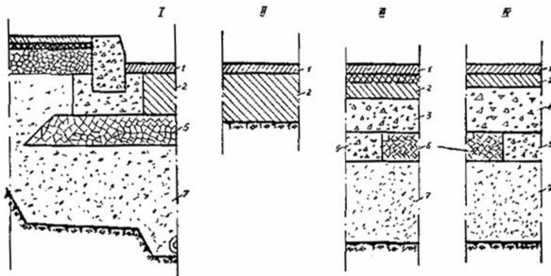
Рис.1. Принципиальные схемы конструкций дорожных одежд с асфальтобетонным покрытием.
